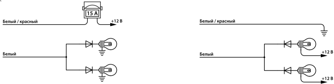
Схема 2. Способы подключения световой сигнализации. Белого и белого/красного проводов в зависимости от требуемой полярности
