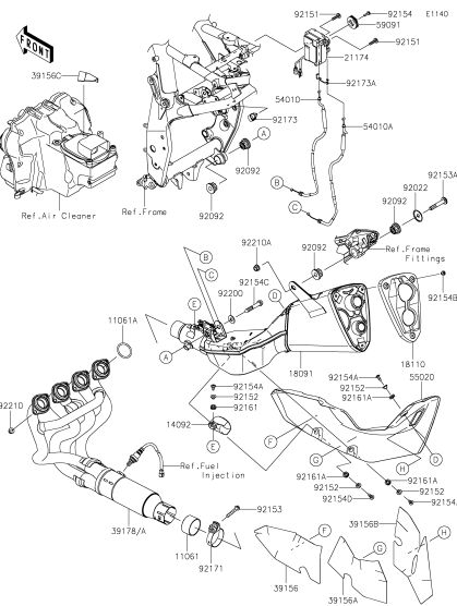
B-7 Muffler(s)
