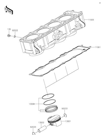
B-5 Cylinder/Piston(s)
