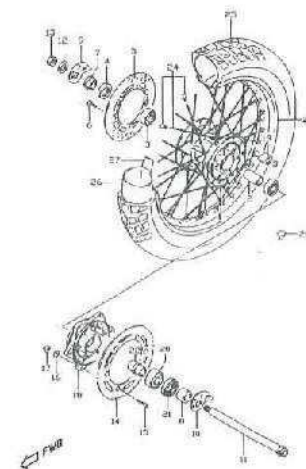
FIG.56 OPTIONAL (I-14)
