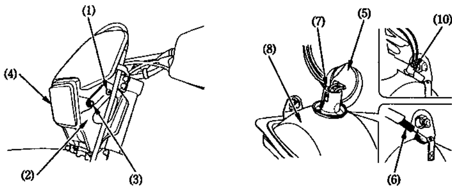
(1) Крепежный болт (2) Корпус фары (3) Болт (4) Передняя фара (5) Резиновый чехол (6) Пружина (7) Разъем (8) Передняя фара (9) Лампа передней фары (10) Разъем (только для модификации ED) (11) Лампа фары габаритного огня (только для модификации ED)
