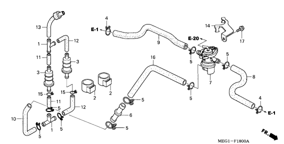
エアージェクションコントロールバルブ
