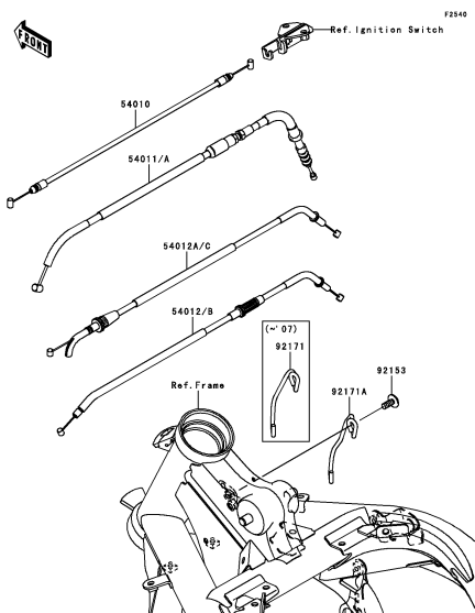
G-3 Cables
