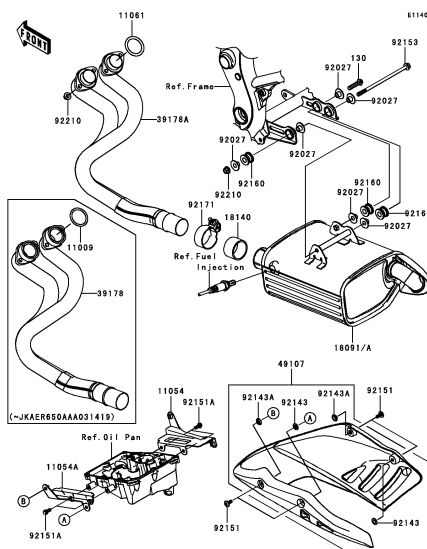
B-7 Muffler(s)
