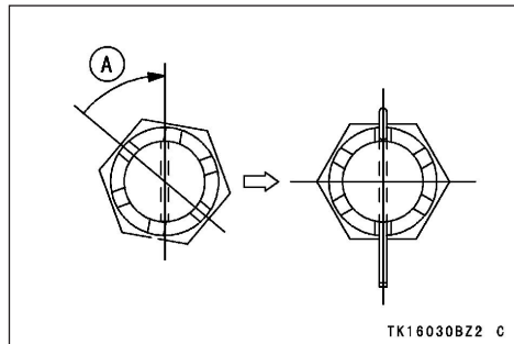
A. Поворот по часовой стрелке
