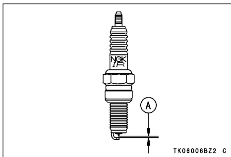
A. Зазор свечи 0.8 – 0.9 мм
