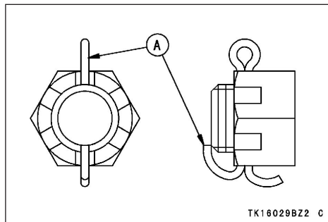
A. Контровочный шплинт
