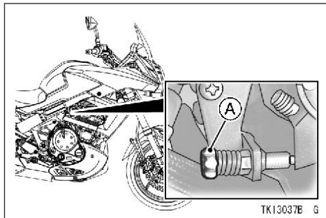
A. Винт регулировки оборотов холостого хода
