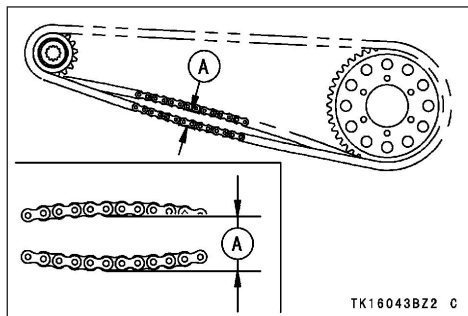
А. Натяжение цепи
