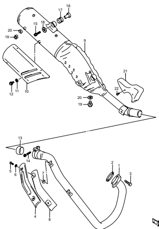
FIG.13 MUFFLER (C-5)
