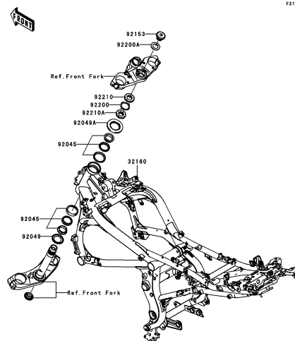
E-4 Frame(A9F)
