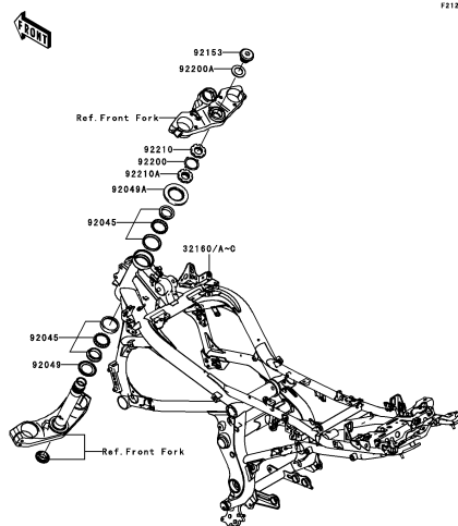
E-3 Frame(A7F/A8F)
