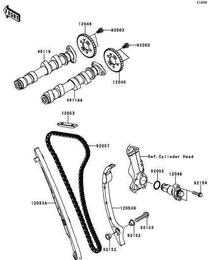
B-9 Camshaft(s)/Tensioner
