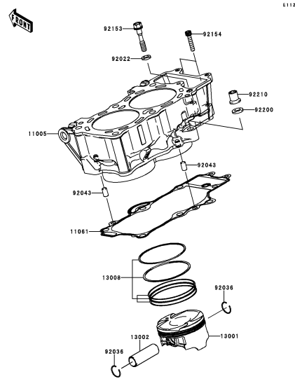
B-5 Cylinder/Piston(s)
