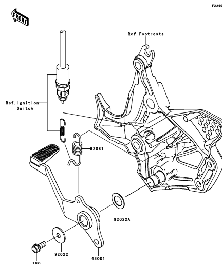
F-4 Brake Pedal
