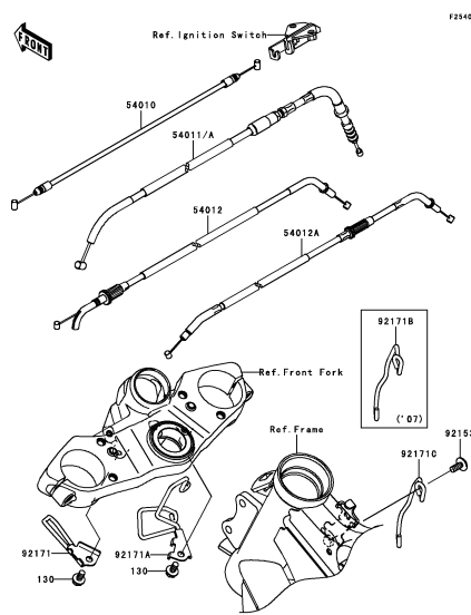
G-7 Cables
