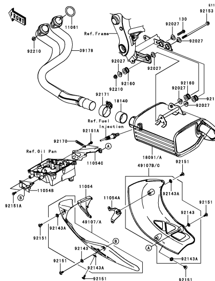
B-7 Muffler(s)
