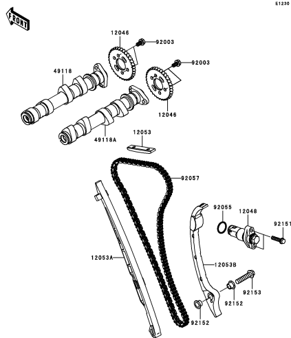
B-9 Camshaft(s)/Tensioner
