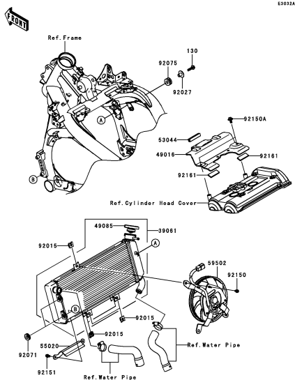
D-9 Radiator(B9F)
