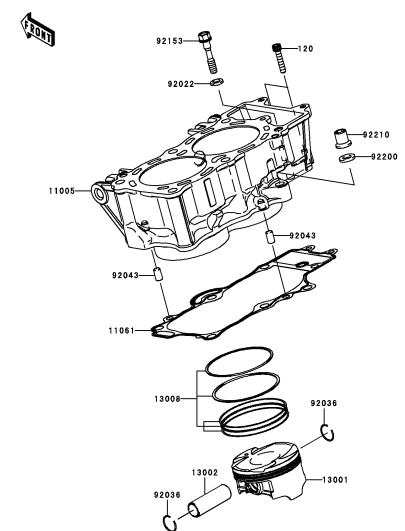
B-5 Cylinder/Piston(s)
