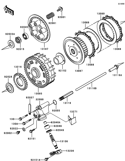
C-3 Clutch
