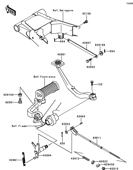
E-14 Brake Pedal
