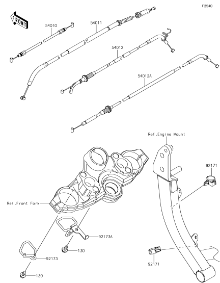
F-14 Cables
