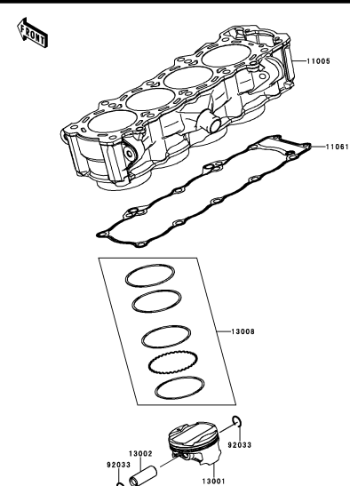
B-5 Cylinder/Piston(s)
