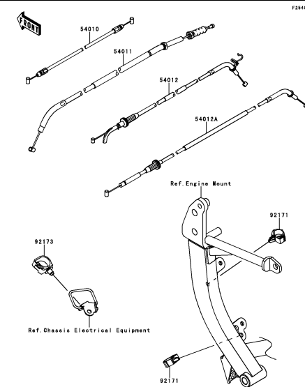
F-14 Cables
