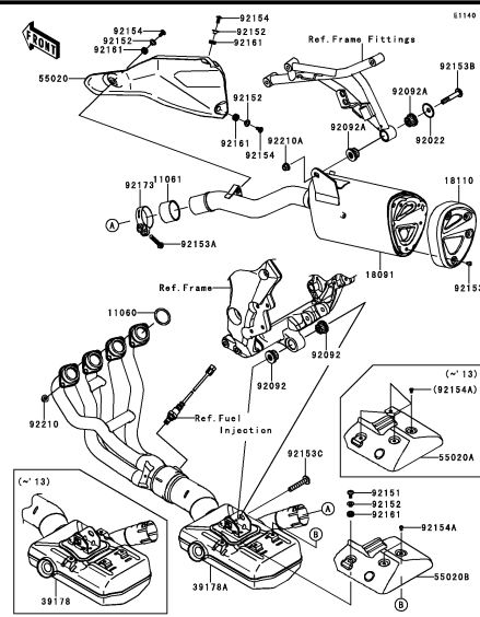
B-7 Muffler(s)
