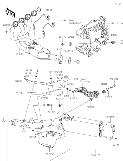
B-6 Muffler(s)
