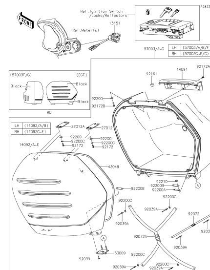
I-5 Saddlebags
