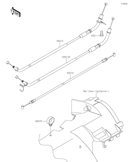
G-8 Cables
