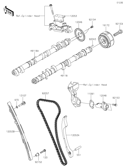
B-9 Camshaft(s)/Tensioner
