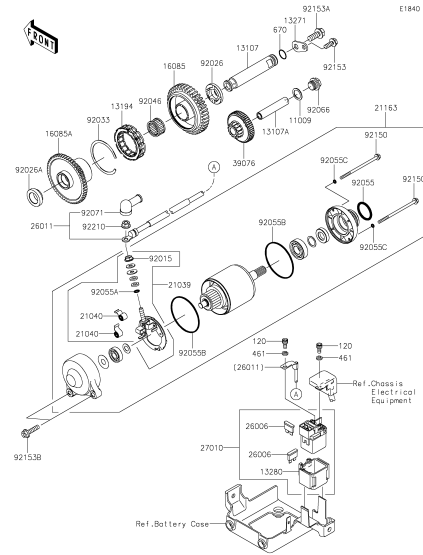
D-4 Starter Motor
