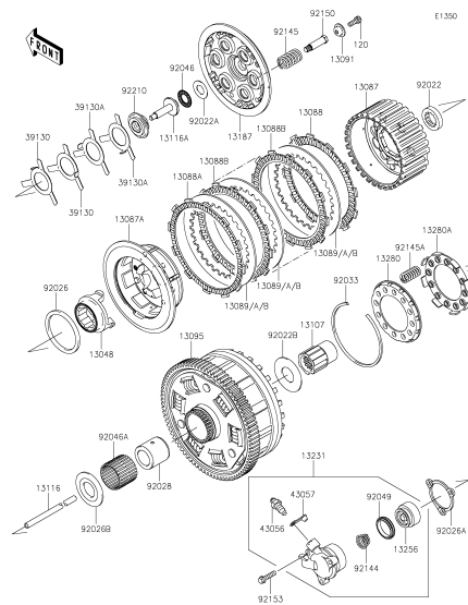
B-13 Clutch(2/2)
