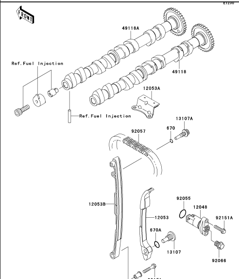
B-9 Camshaft(s)/Tensioner
