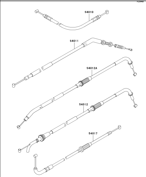
F-14 Cables
