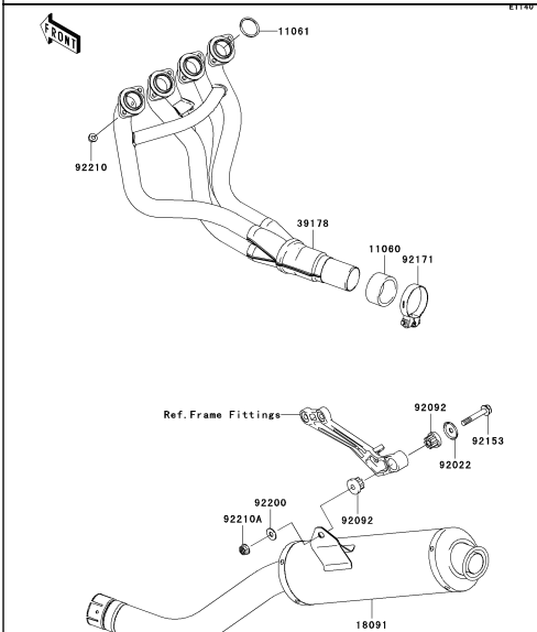
B-7 Muffler(s)
