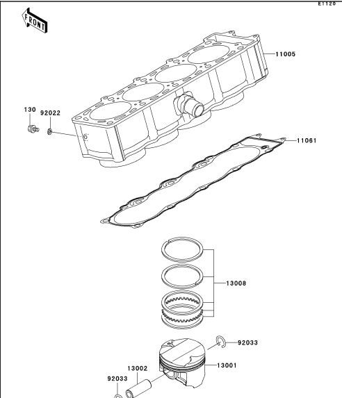
B-5 Cylinder/Piston(s)
