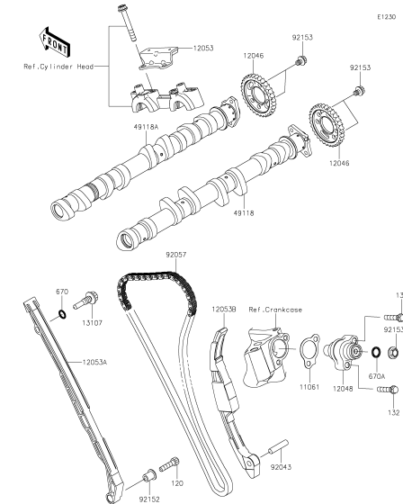
B-11 Camshaft(s)/Tensioner
