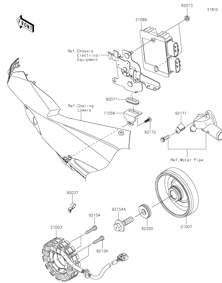
D-4 Generator
