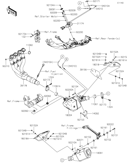
B-7 Muffler(s)
