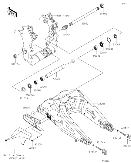
E-6 Swingarm
