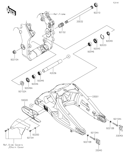
E-6 Swingarm
