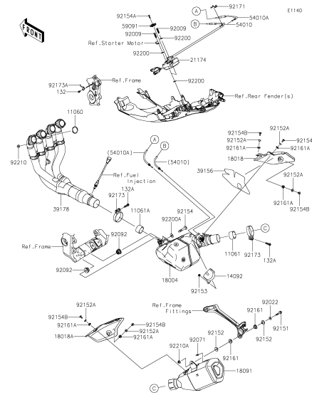
B-7 Muffler(s)
