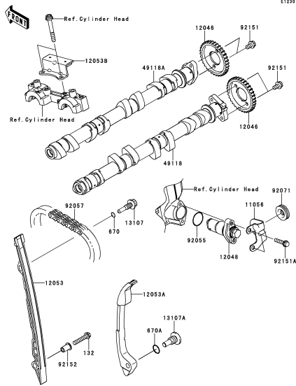
B-9 Camshaft(s)/Tensioner
