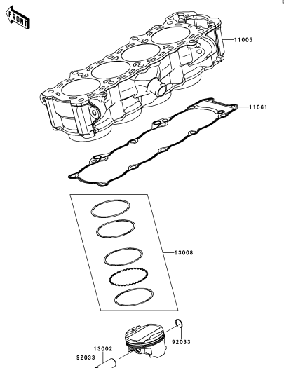
B-5 Cylinder/Piston(s)
