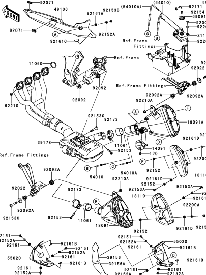
B-7 Muffler(s)
