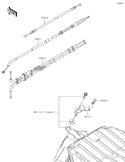
G-3 Cables
