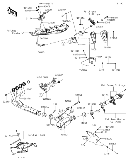
B-7 Muffler(s)
